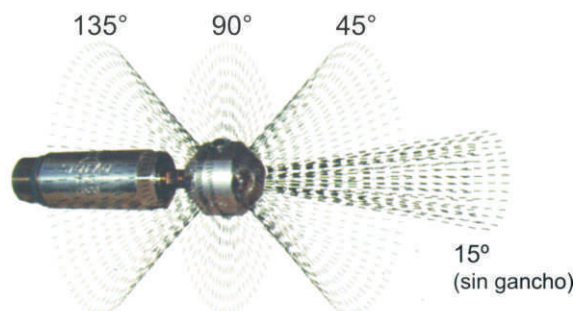
Cabezal con porta toberas RPT 043-P2-7
